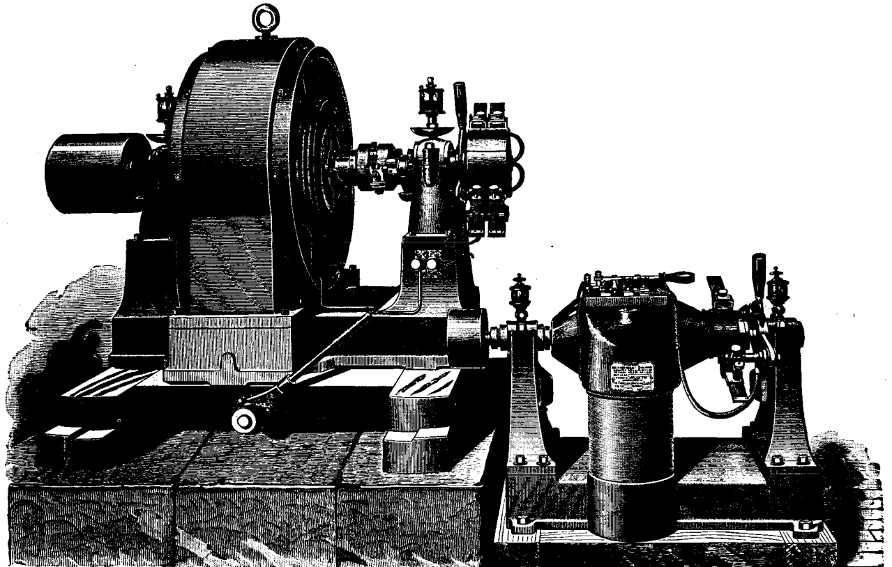
Dinamo y excitador sistema incandescente de Thomson Houston
