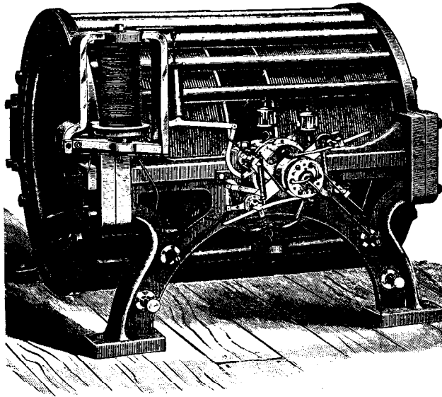
Dinamo sistema arco de Thomson Houston
