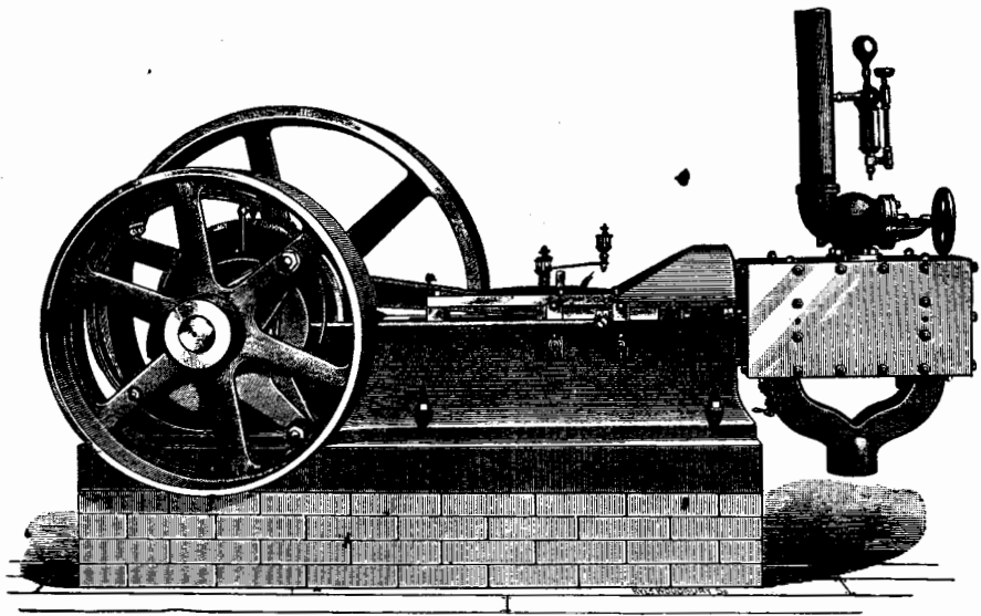
UNO DE LOS MOTORES.
